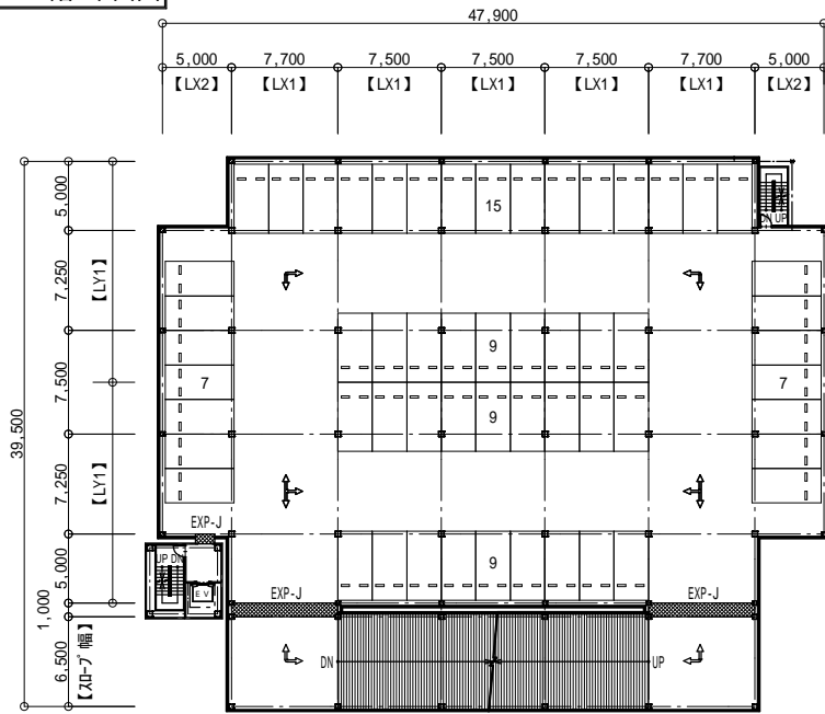
2～6階 平面図
